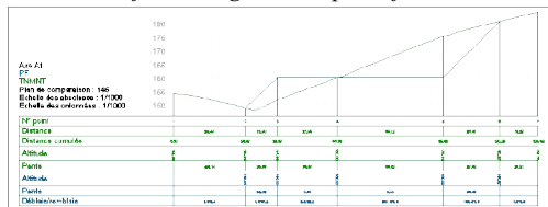
Profil en long sur une plate-forme
